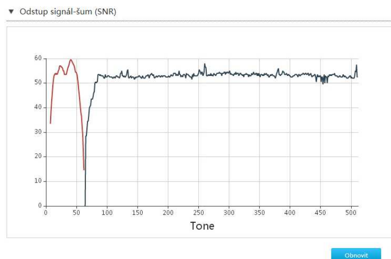
Obrázek 112 Odstup signál šum (SNR)
