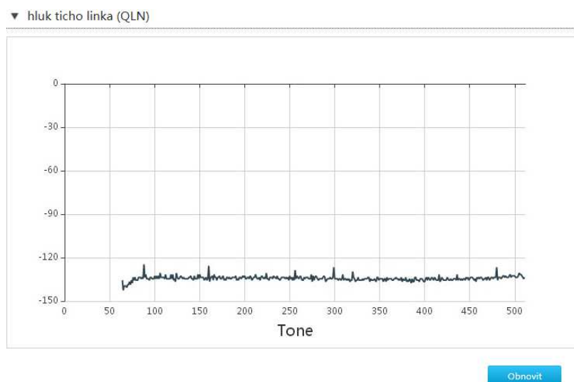
Obrázek 111 Hluk ticho linka (QLN)
